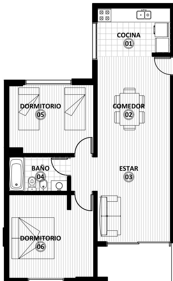
PLANTA TIPO-DEPARTAMENTO 02
